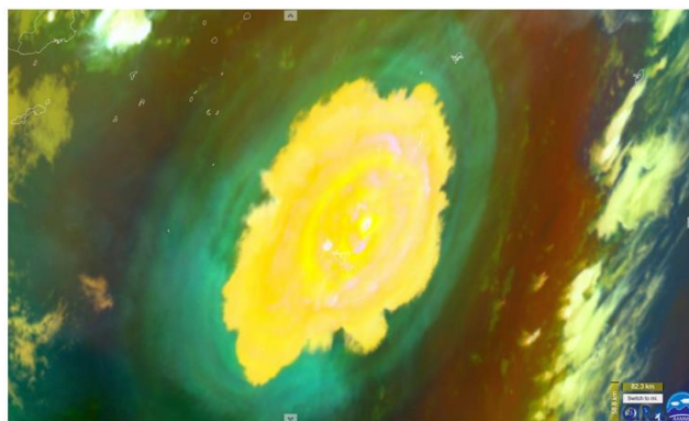
Figure 22 - Himawari-8 Airmass RGB, 15 janvier 05:10 TU. Crédit : CIRA 28 .
